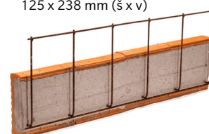
Porotherm KP Vario 200-350 (rozmery prekladu v reze: 70 x 238 mm)
