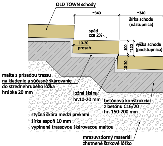
Vzorový rez osadenia na monolitický betónový podklad
