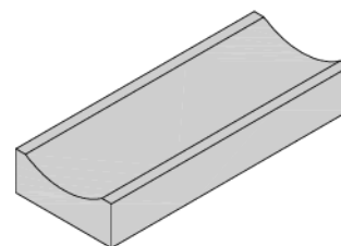
Odvodňovací žlab 50/20/8 cm Prehĺbenie 2,5 cm
