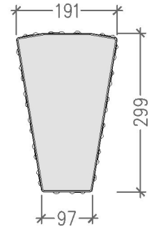
10 x 20 x 30 cm klinový prvok
