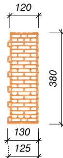
Porotherm 38 Profi Dryfix 1/2 K (1/2 K = polovičná koncová)
