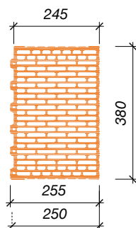
Porotherm 38 Profi Dryfix K (K = koncová)
